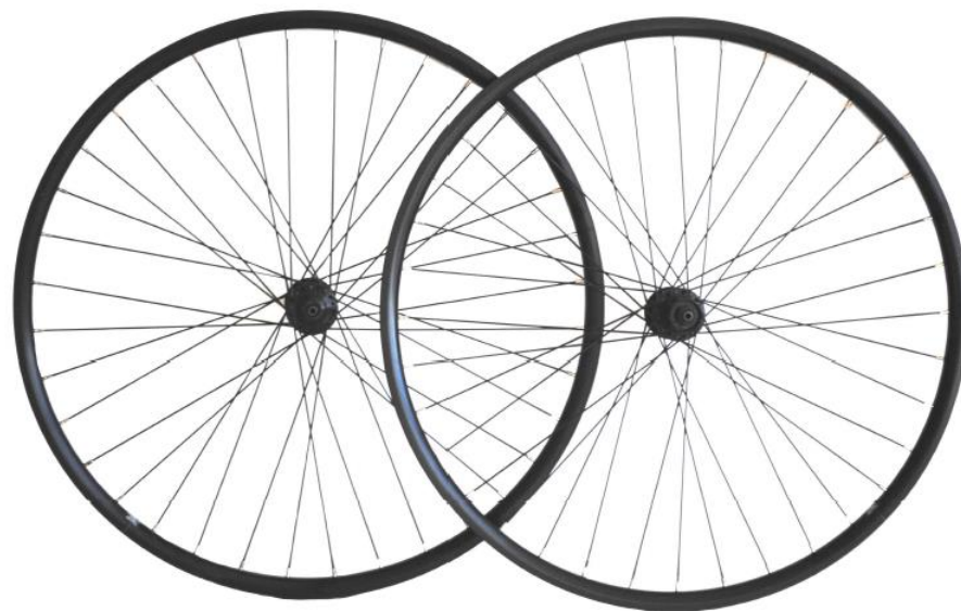
Rodas MISSION 27,5 ER 20 Cubo Shimano 36 F. REF.: 40.340.6 – Par
