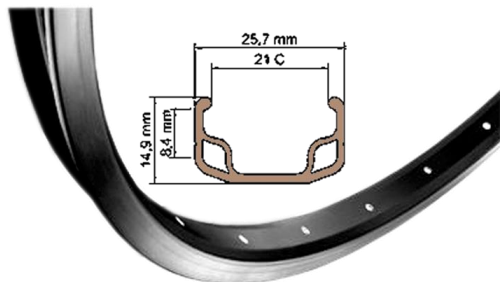
Aro 24" Mach 1 M110 Raw 36 Furos Preto
